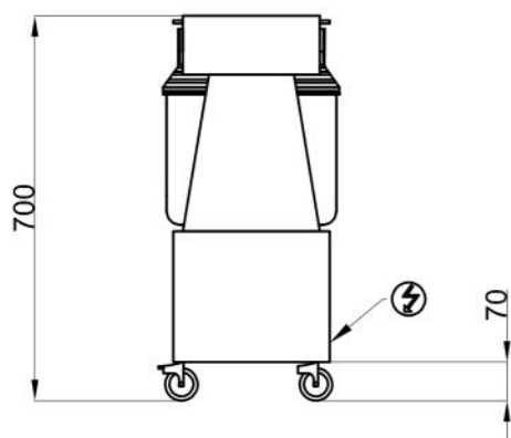
VISTA DIETRO
