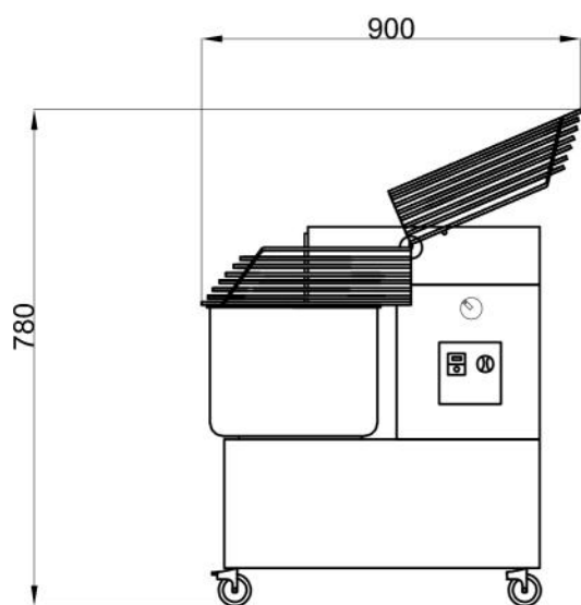
VISTA LATERALE
