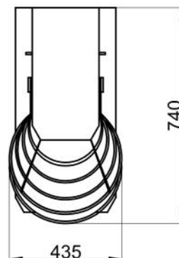
VISTA DALL'ALTO
