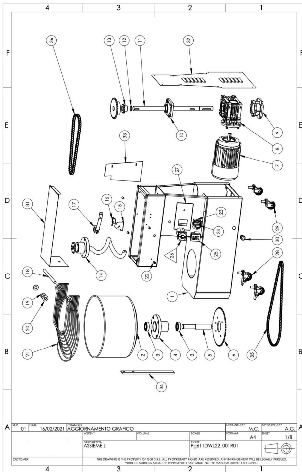
Fig. 10-11. L22 / L33 / L42 / L53 / L62 assembly
